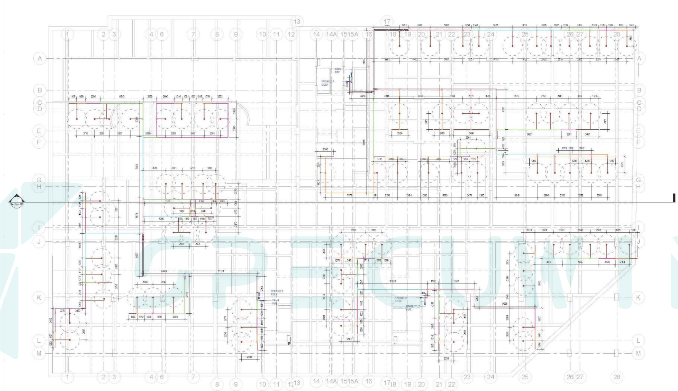
1 B3 PLAN 1:150
